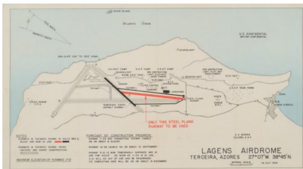
Figura 14 - Planta da pista das Lajes e previsão da conclusão dos trabalhos de expansão. Julho de 1944.
