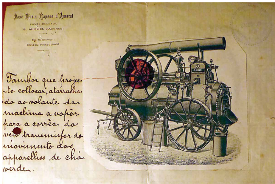
2 – Projeto de tambor para máquina a vapor aplicada à produção de chá verde, 1914 (UAc: BAM: ARA)
