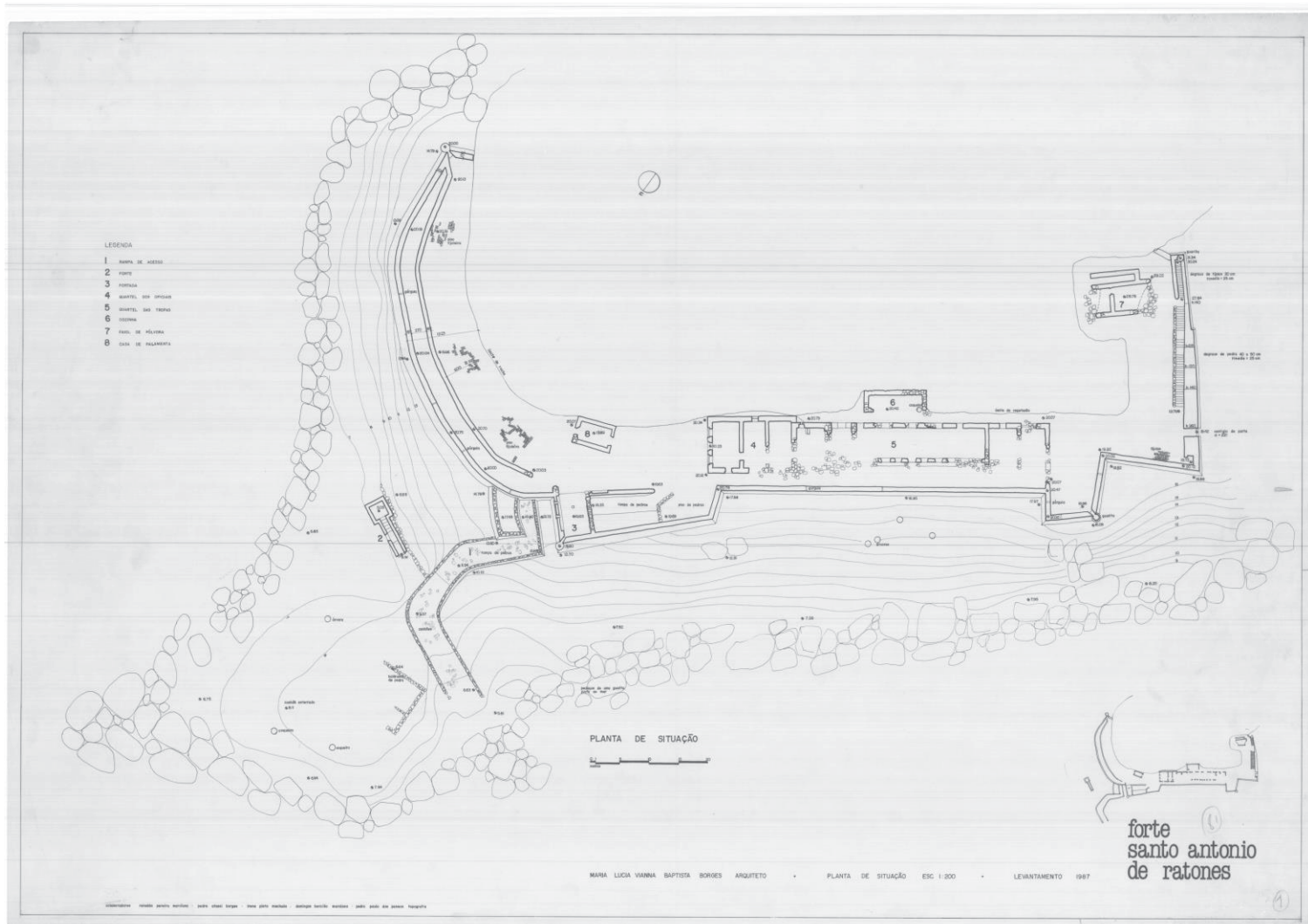
14 - Planta Geral de situação, escala 1:200, que integra o levantamento cadastral das estruturas arruinadas da Fortaleza de Santo Antônio de Ratores, realizado em 1987.
