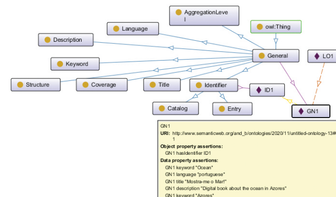
Fig. 2 Exemplo de ABox usada para armazenar metadados
