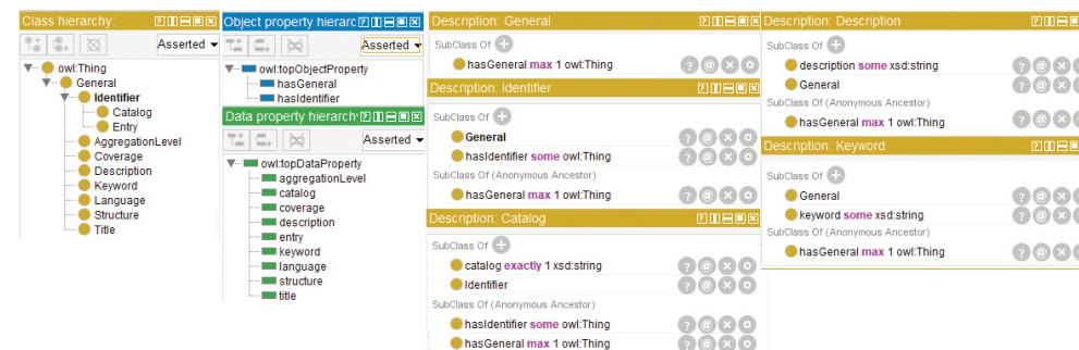
Fig. 1 TBox dos metadados de OAs para a categoria Geral
