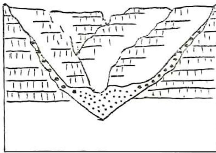
Kerbtal
