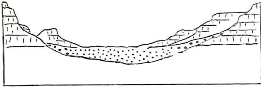
Kehltal
