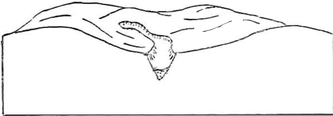
Muldental
