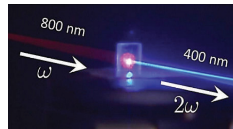
Fig. 3 - Geração de segundo harmónico. Adaptado de https://www.osti.gov/servlets/purl/1510171
