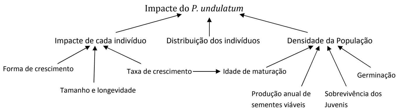
Figura 3.2 - Factores determinantes para avaliação dos impactos do P. undulatum .
