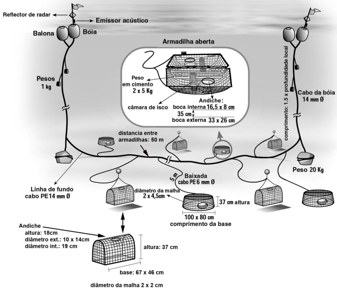
Figura 4. Esquema da arte utilizada na prospecção de caranguejos e camarões de profundidade nos Açores. Nos lances dirigidos a camarão foram alternados covos do fundo com covos alvoraços do fundo cerca de 5 m, utilizando bóias de profundidade.
