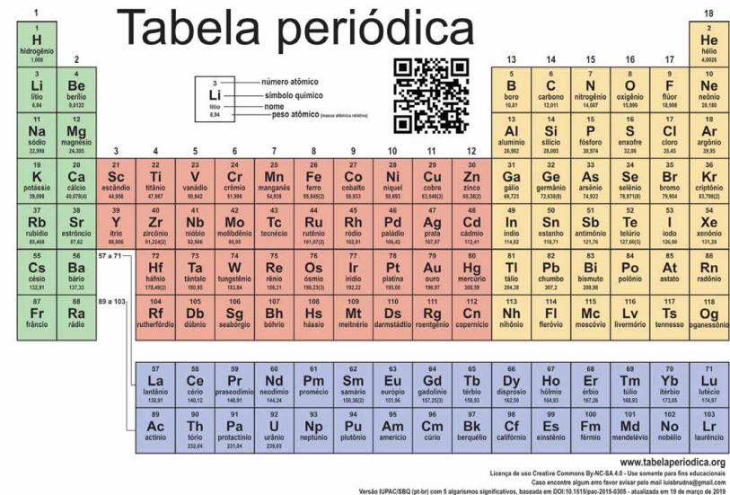
Figura. 2: Tabela Periódica dos Elementos Químicos atual ( https://www.tabelaperiodica.org/imprimir/ ).
