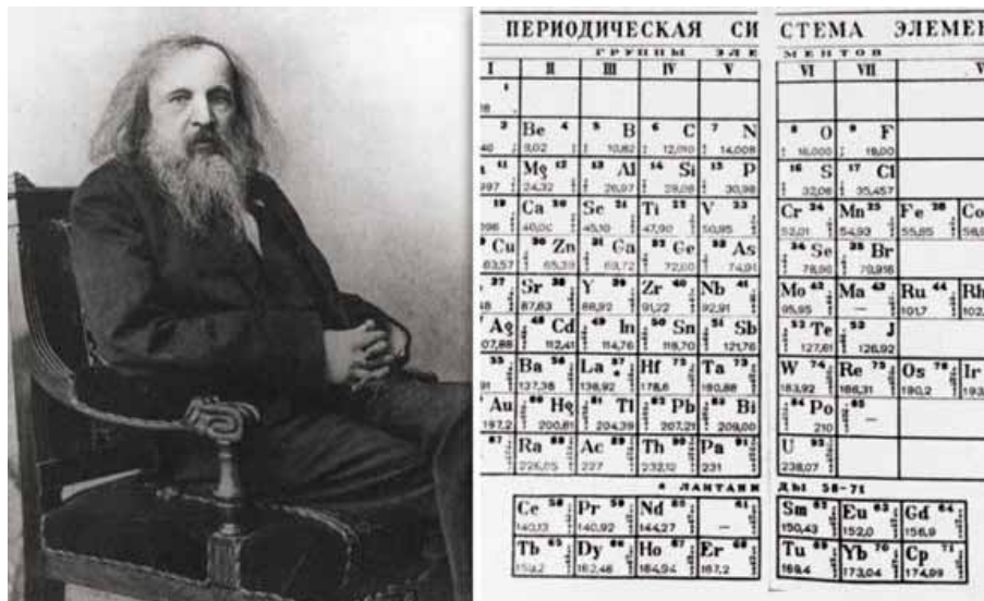
Figura. 1: Tabela Periódica dos Elementos Químicos publicada por Dimitri Mendeleev em 1869 ( https://www.gettyimages.pt/ )
