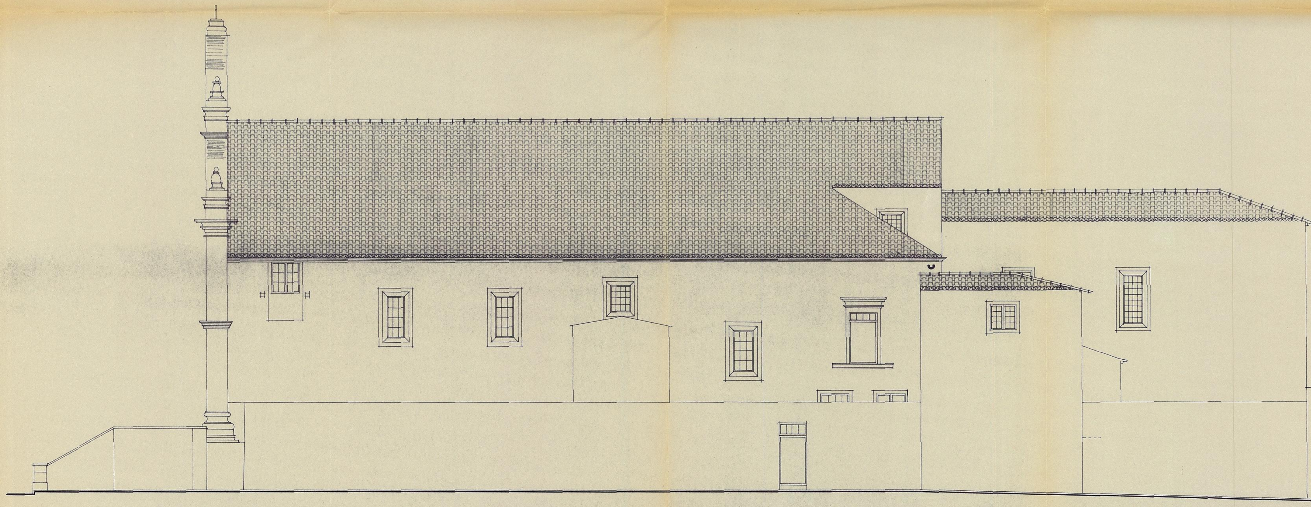
ALÇADO LAT. DIREITO
